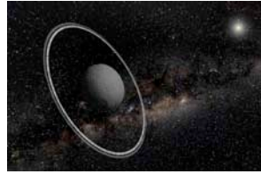
10199 Chariklo et son système d'anneaux. © L. Maquet / Observatoire de Paris / LESIA
